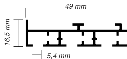
Rozměry trojkolejničky pro japonské posuvné stěny
