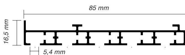
Rozměry pětikolejničky pro japonské posuvné stěny
