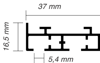
Rozměry dvojkolejničky pro japonské posuvné stěny
