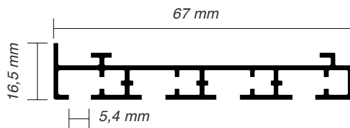
Rozměry čtyřkolejničky pro japonské posuvné stěny
