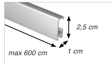
Rozměry kolejničky Gerika
