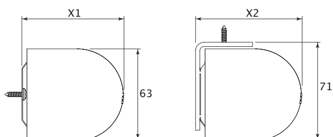
Rozměry rolety KC v mm
