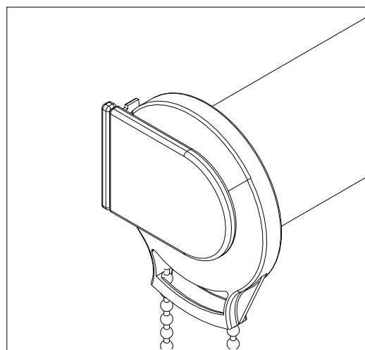
Detail Rolety OS - montovaná na zeď
