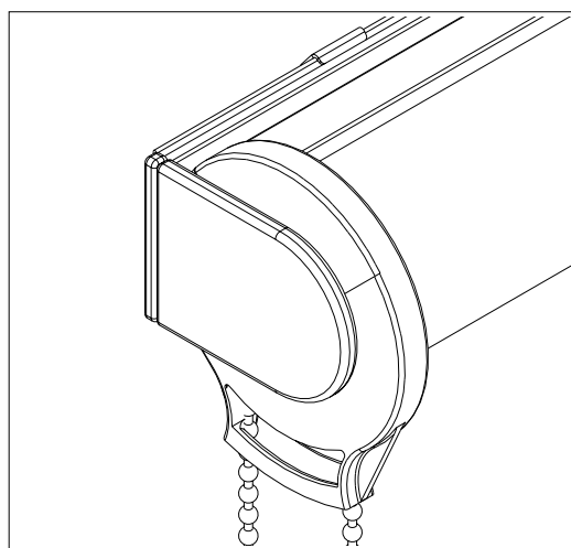
Detail Rolety OMP - montovaná přes montážní profil
