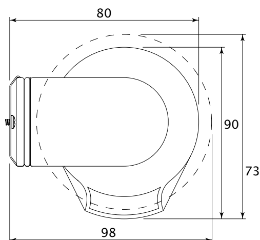
Rozměry rolety OMP
