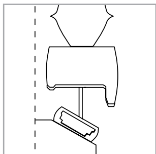
Upravený dolní profil pro šikmou zasklívací
