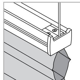
Magnetický uzávěr zajišťuje dodatečné uchycení v horní poloze
