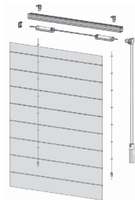
Komponenty římských rolet
